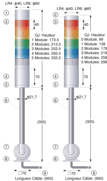
Montage C [QJ] Montage Tube avec Support Orientable et Câble (02: 24V DC)
