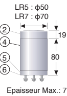
Montage A [WT] Montage Direct / Bornier Débrochable (Base)
