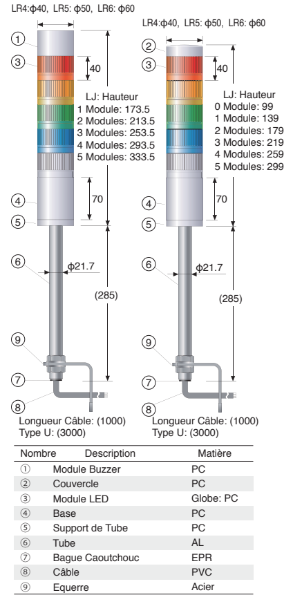
Montage B [LJ] Montage Tube avec Equerre et Câble (01: 12V DC/ 02: 24V DC)
