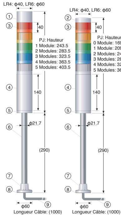
Montage A [PJ] Montage Tube avec Support Circulaire et Câble (M2: 100V - 240VAC)
