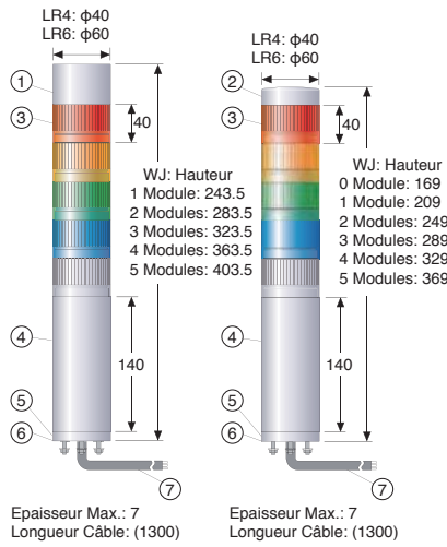
Montage A [WJ] Montage Direct/Câble (M2: 100V - 240VAC)
