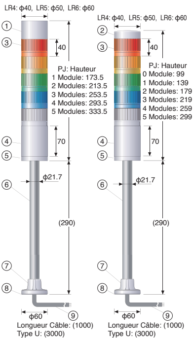
Montage A [PJ] Montage Tube avec Support Circulaire et Câble (01: 12V DC/ 02: 24V DC)
