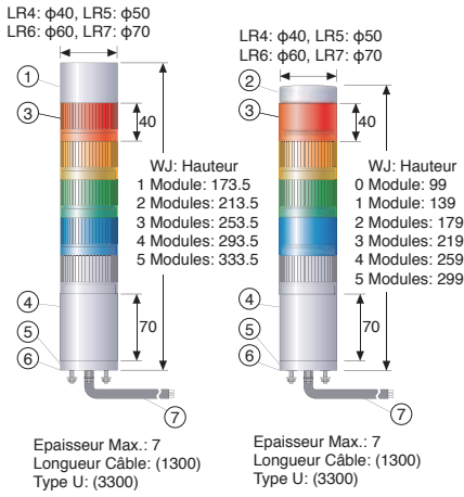
Montage A [WT] Montage Direct / Bornier Débrochable (Base)
